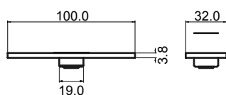
Platina de instalación
