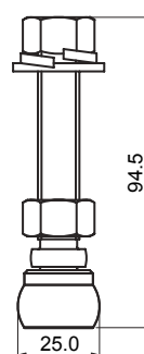
Guía Inferior 25 mm
