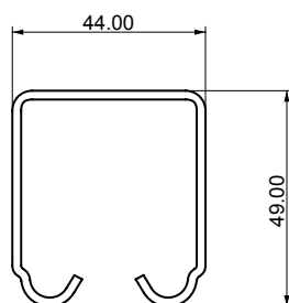
Riel U-300
