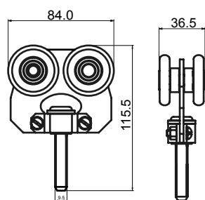
Carro DN 300 HD
