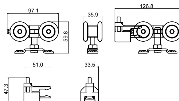
Carro DN 150
