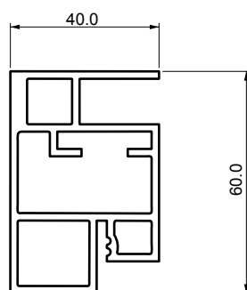
Perfil marco perimetral
