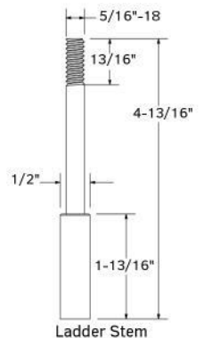
Ladder Stem
