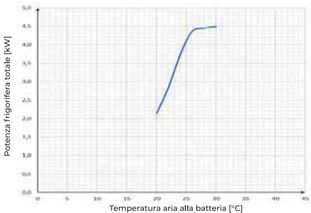
RESA FRIGORIFERA (3)
