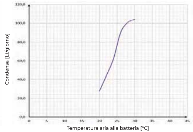
CAPACITA' DI DEUMIDIFICA (2)
