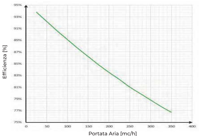
EFFICIENZA TERMICA (1)
