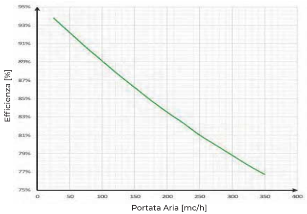
EFFICIENZA TERMICA (1)
