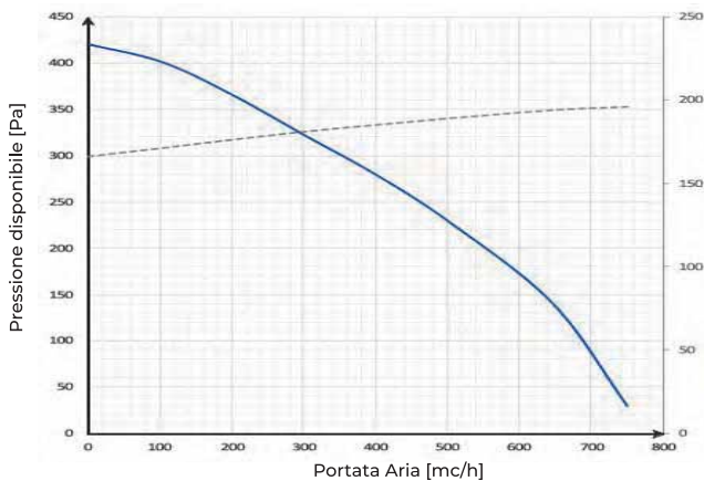
PRESTAZIONI AREAULICHE PORTATA TOTALE
