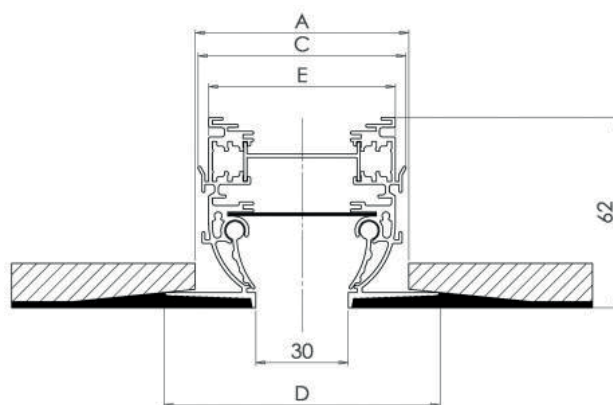
Diffusore lineare a scomparsa con feritoia da 30 mm.
