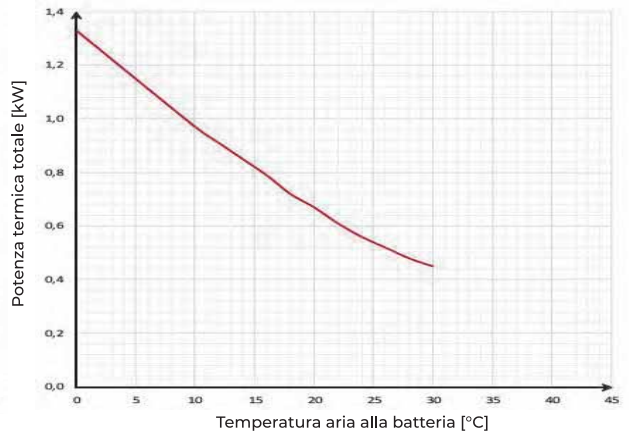
RESA TERMICA (4)
