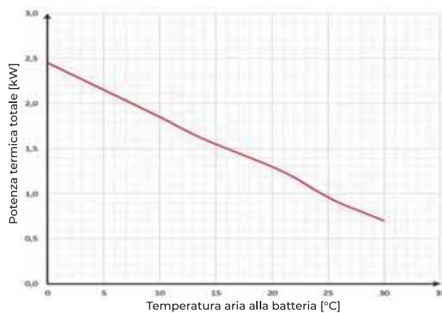
RESA TERMICA (4)
