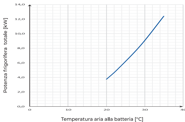
RESA FRIGORIFERA BATTERIA IDRONICA (4)
