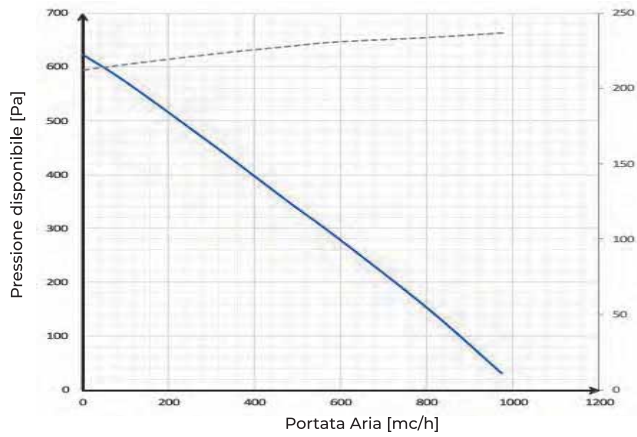
PRESTAZIONI AREALICHE PORTATA TOTALE
