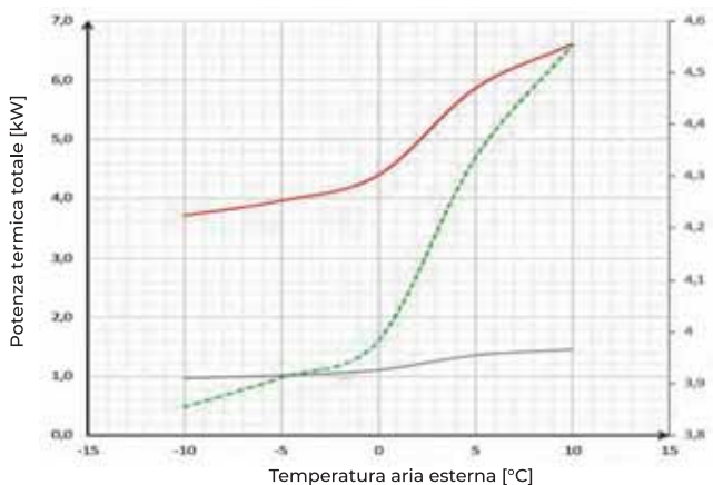
POTENZA TERMICA (3)
