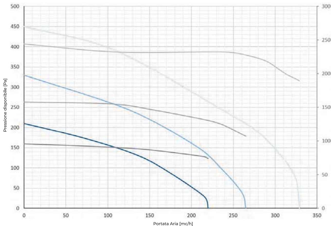
PRESTAZIONI AREAULICHE
