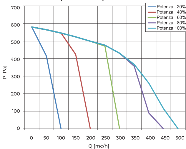
Curve caratteristiche ventilatore estrazione SALUS H-C 450: prevalenza disponibile
