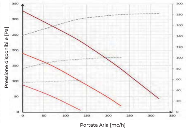
PRESTAZIONI AREALICHE ESPULSIONE
