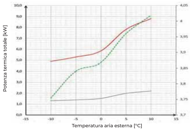
POTENZA TERMICA (3)
