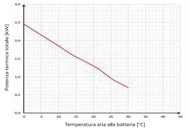
RESA TERMICA (4)
