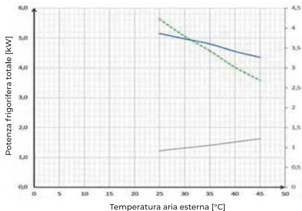
POTENZA FRIGORIFERA (4)
