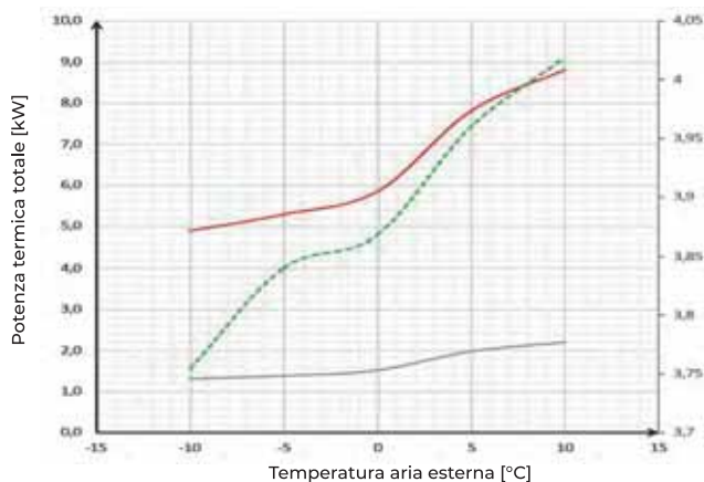
POTENZA TERMICA (3)
