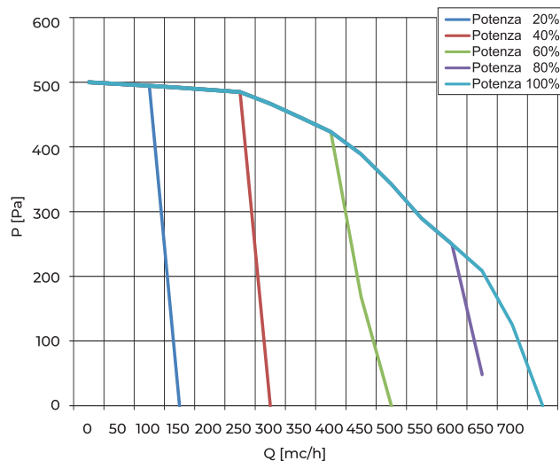
Curve caratteristiche ventilatore mandata SALUS H-C 450: RICIRCOLO
