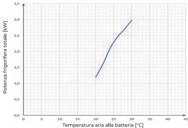
RESA FRIGORIFERA (3)
