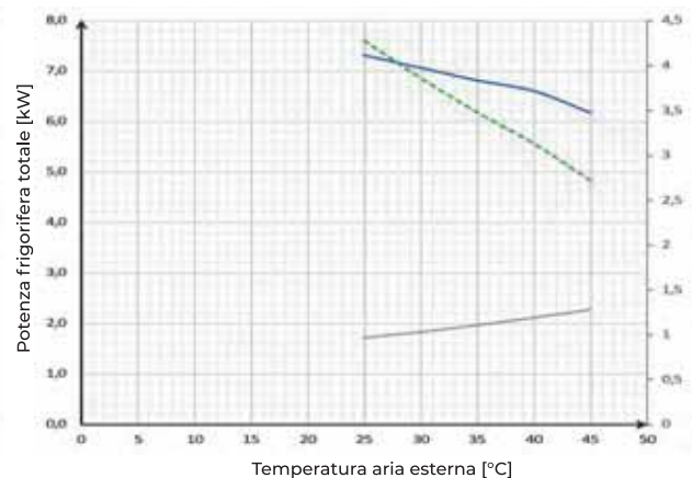
POTENZA FRIGORIFERA (4)
