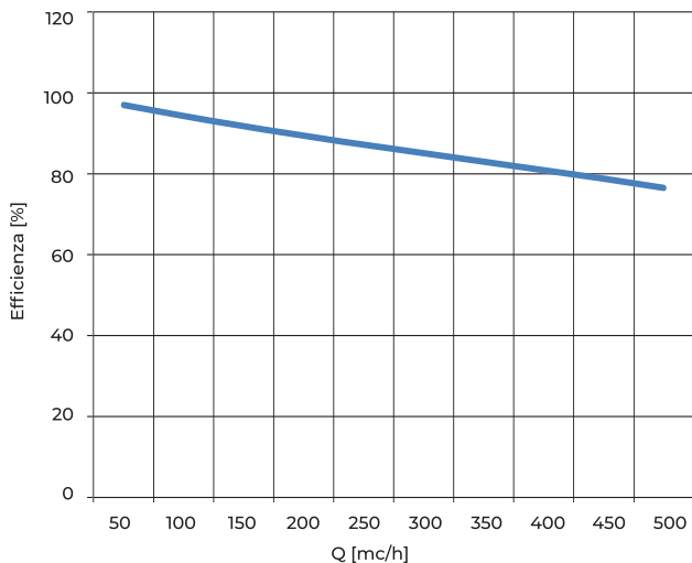
Efficienza SALUS H-C 450
