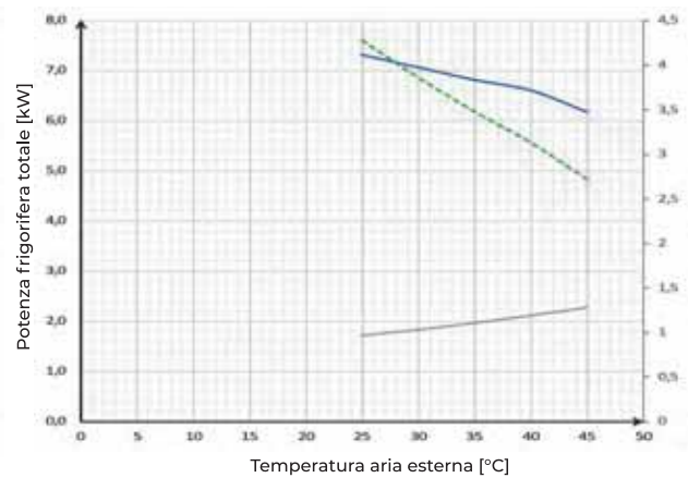
POTENZA FRIGORIFERA (4)
