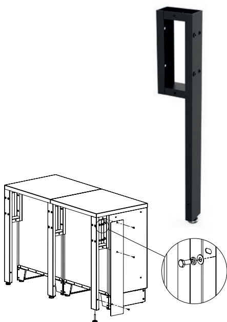
BUNKER Support de fixation modulaire pour plan de travail, 61cm
