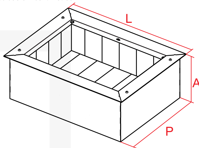
Figura 7 - Dimensões.
