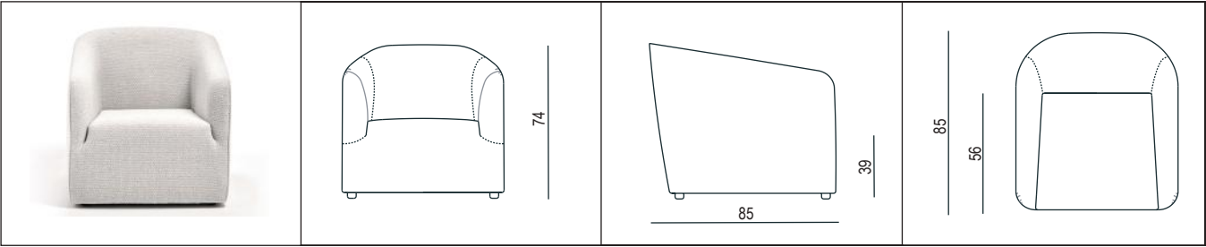
BUTACA TAPIZADA FIJA NON REMOV. ARMCHAIR 74X85
