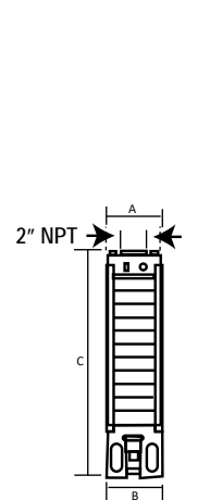
Acoplamiento NEMA 4"
