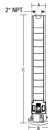
Acoplamiento NEMA 6"
