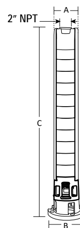
Acoplamiento NEMA 6"
