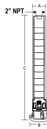
Acoplamiento NEMA 6"
