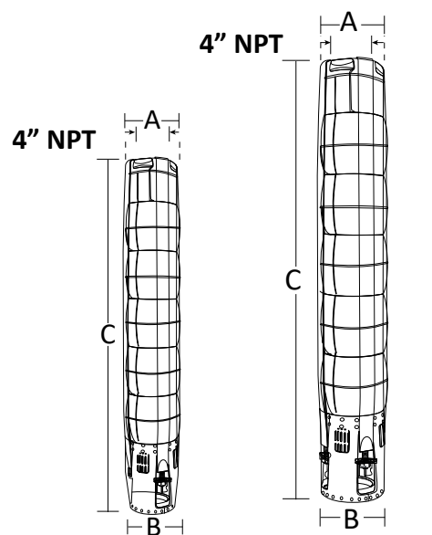
Acoplamiento NEMA 4"
