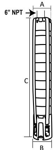
Acoplamiento NEMA 8" Fin 2
