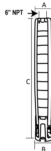
Acoplamiento NEMA 6" Fin 1
