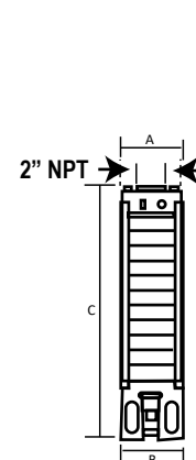
Acoplamiento NEMA 4"
