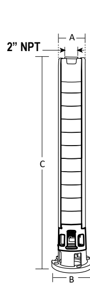
Acoplamiento NEMA 6"
