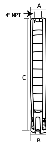
Acoplamiento NEMA 4" Fig. 1
