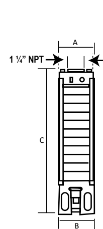
Acoplamiento NEMA 4" Fig. 1
