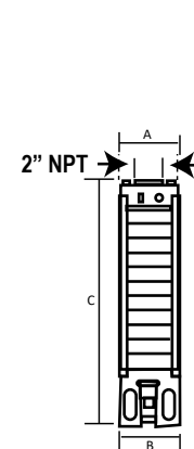
Acoplamiento NEMA 4" Fig. 1
