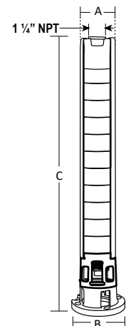
Acoplamiento NEMA 6" Fig. 2
