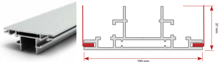
Profil, doppelseitig, freistehend, 100 mm IS-9665
