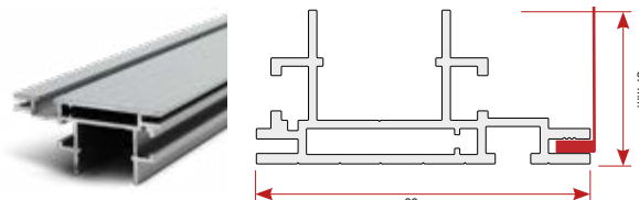
Profil, einseitig, eingebaut, 80 mm IS-9664
