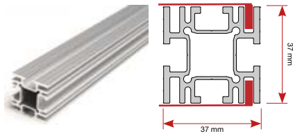
SYSTEM-RAHMEN Profillängen 3100 mm IS-9097
