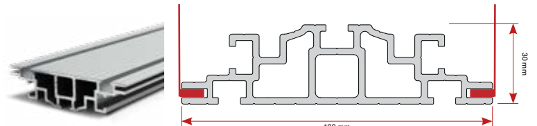
Profil, doppelseitig, eingebaut, 120 mm IS-9332
