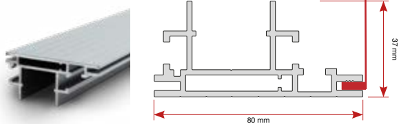
Profil, einseitig, Wandmontage, 80 mm IS-9647
