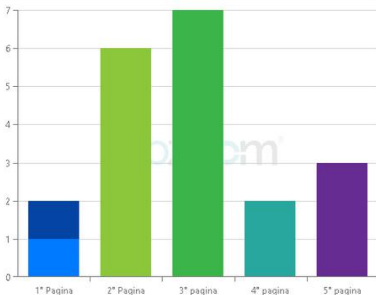
Distribuzione keyword
