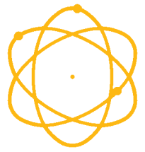
원자
