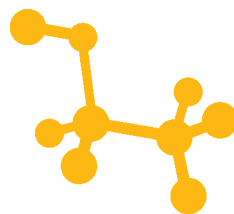
분자 구조
