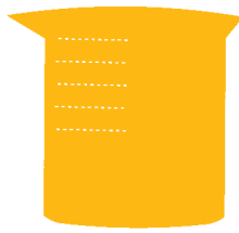
비이커
