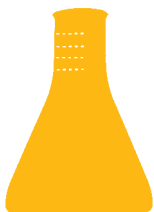
플라스크
