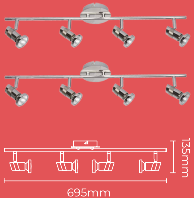
Aplique PARTY 4 Art.: C090/4
