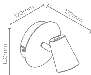
Aplique SONATA 1 Art.: C955/1 NT
