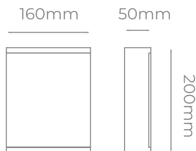
Aplique SEÑAL Art.: B5790
