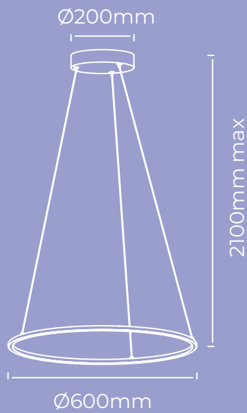
Colgante LAZO 60 Art.: CTL910006041
