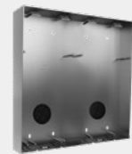
Opbouwdoos met regenkap voor panelen met infomodule 313 (B) x 320 (H) x 50 (D) mm
