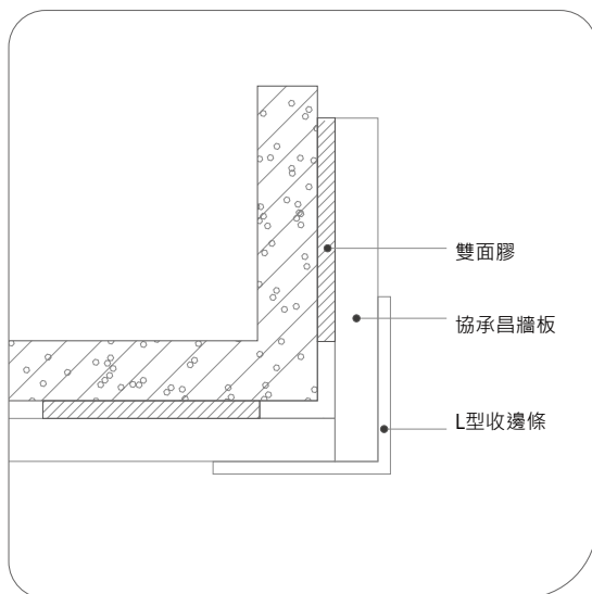
牆板窗台陽角收口大樣圖
