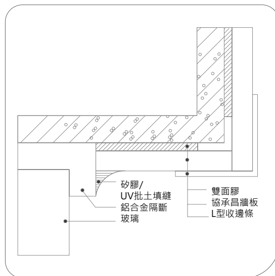
牆板窗台窗戶節點大樣圖
