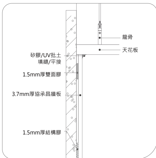
牆板與天花板交接大樣圖
