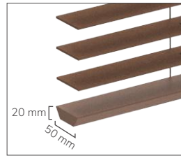
Bottom Bar
