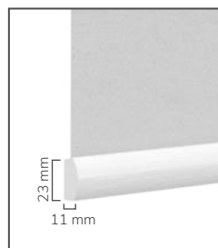
Bottom Bar
