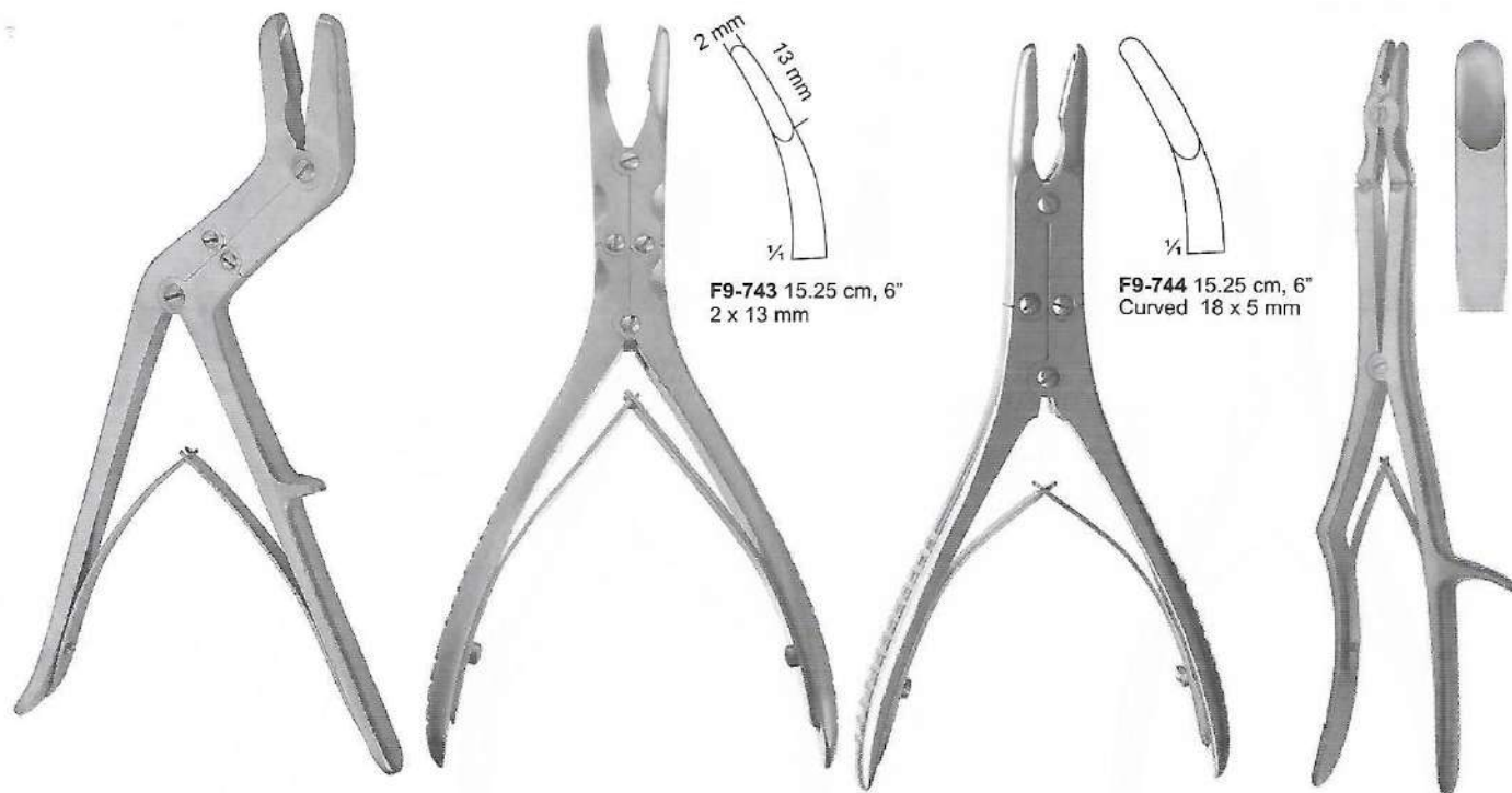
Hakansson Bone Rongeur F9-742 20cm, 8"
