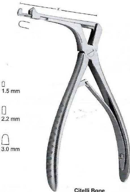
Citelli Bone Ear Rongeurs F10-139 17 cm 6 3/4" X = 60 mm
