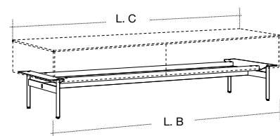
Basamento P 38 cm - 15"
