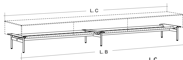
Basamento con sostegno centrale P 38 cm - 15"
