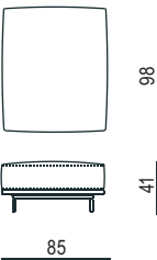
POUF OTTOMAN 85 X 98
