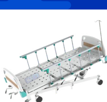
Cama múltiples posiciones (3 manivelas)
