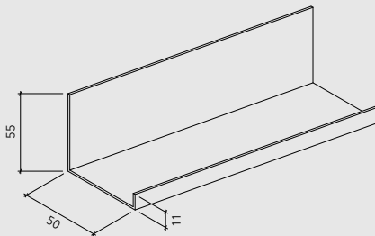
PERFIL MULLION
