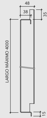
CORTE B
