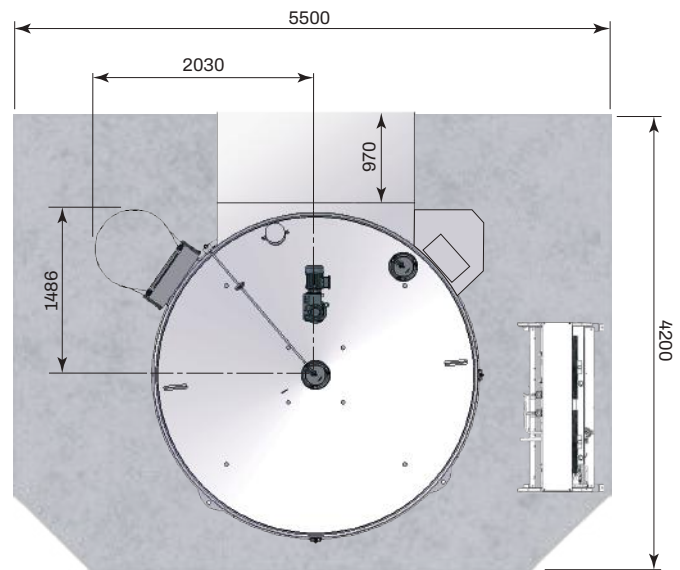
Dalle béton pour silo 3.0
