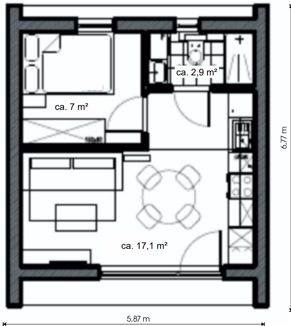
Begane grond
