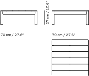
LOUNGETISCH, H27
