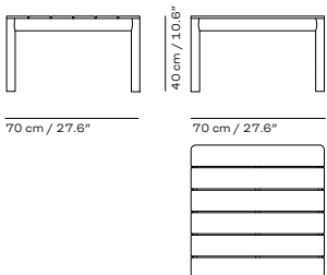
LOUNGETISCH, H40
