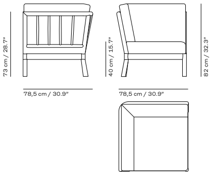
ECKMODUL
