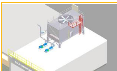
NUEVO DINAMÓMETRO PARA PRUEBA DE MOTORES DIESEL MULTIMARCA HASTA 6000 HP
