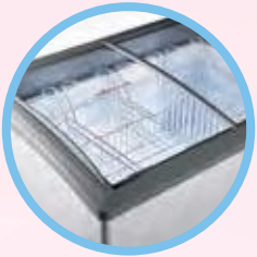
Lid & Baskets detail
