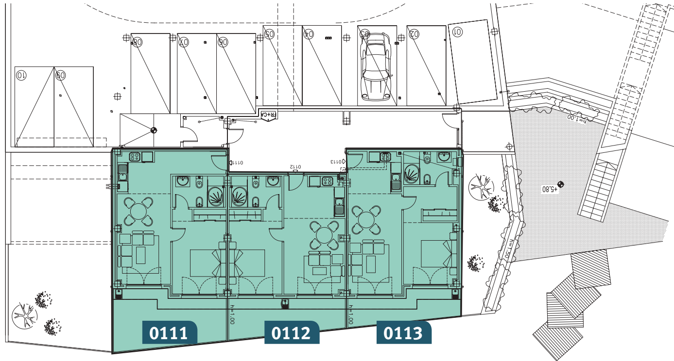
Vooranzicht 2
