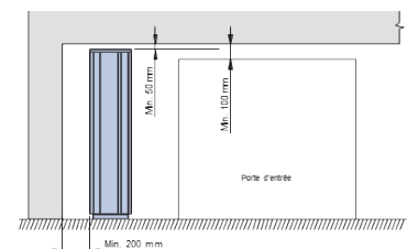
Sez. verticale
