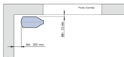
Sez. orizzontale
