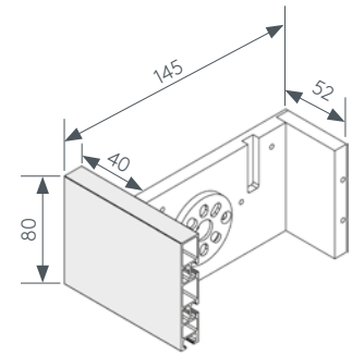
Abb. Wandträger
