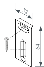
Abb. Montageplatte
