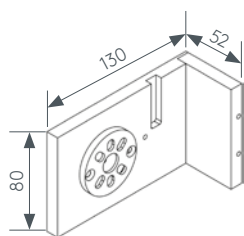
Abb. Wandträger
