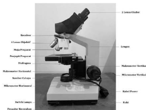
Gambar Bagian-bagian Mikroskop Binokuler (Dok. Pribadi)
