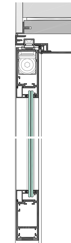
LZS48-5-42SL mit flächenbündiger Aluminium Rahmentür ART42
