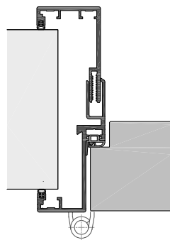
UST56-5-70SL mit Türblatt 70mm
