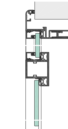
EURORF30-5-8G mit Ganzglastür 8mm und Oberlicht, Kämpfer KLF30-35
