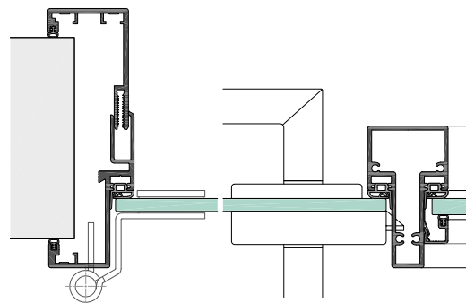
UST48-5-8G mit Ganzglastür, Pfosten KST48 und Glasseitenteil
