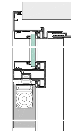
UST48-5-42S mit Türblatt 42mm, Oberlicht und Kämpfer KLS48-20 und ITS
