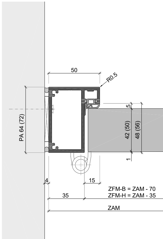
BS48-5-42S Blockzarge, einteilig, mit stumpf einschlagendem Türblatt
