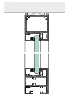
BFF30-5-8G Festverglasung mit Kämpfer KLF30-20
