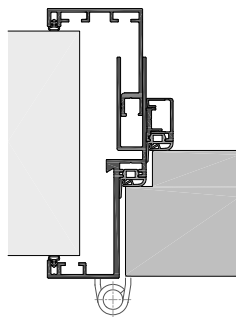
EUROKS56-5-70SL-ZAP Doppelfalzzarge mit Türblatt 70mm
