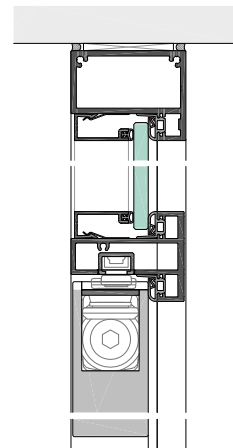
BS48-5-42S Türblatt 42mm, Kämpfer KLS48-20 und Oberlicht, mit ITS
