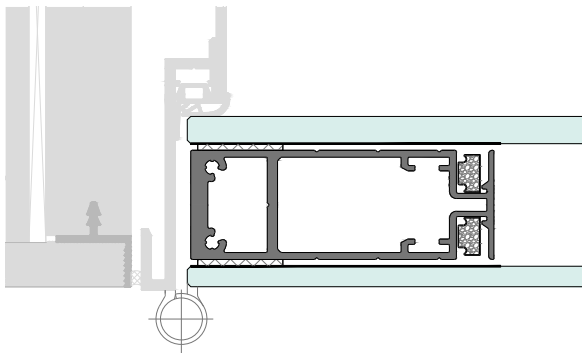
Glasverbundtür GVT50 mit Aluminiumzarge FZ556
