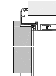
EURORF30-5-42F mit gefälztem Türblatt 42mm
