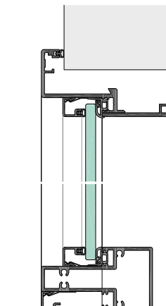
USTB48-5-8G Festverglasung mit Kämpfer KST48
