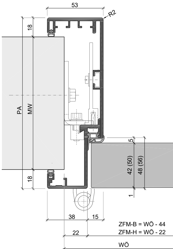
USTB48-5-42S Umfassungszarge mit stumpf einschlagendem Türblatt 42mm
