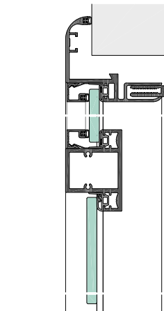
URF30-5-8G mit Ganzglastür 8mm und Oberlicht, Kämpfer KLF30-35
