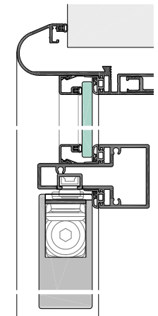
EUROFIS48-5-42S mit Türblatt 42mm und Oberlicht, Kämpfer KST48 sowie ITS
