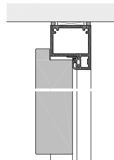
BF30-5-42F mit Türblatt gefälzt
