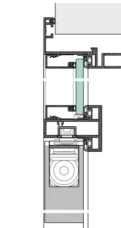
EUROKS48-5-42S mit Türblatt 42mm und Oberlicht, Kämpfer KLS48-20 sowie ITS
