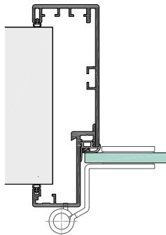
USTB48-5-8G mit Ganzglastür 8mm
