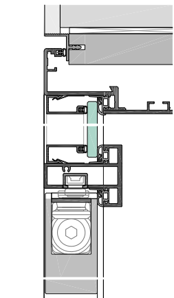
USTB48-G-5-42S mit Grundzarge, Kämpfer KLS48-20, Oberlicht und integriertem Türschließer
