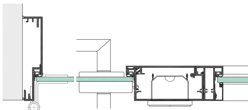
LZSB48-5-8G mit Ganzglastür, Pfosten KLS48-20, Türterminal TTM und Glasseiteenteil
