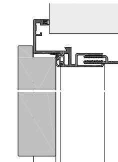
UNF30-5-42F mit gefälztem Türblatt
