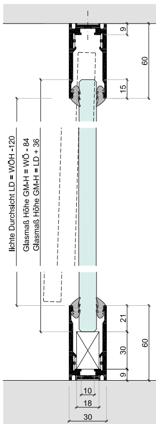
Glasmontage / Glasbemessung nach statischen Erfordernissen (bauseits)
