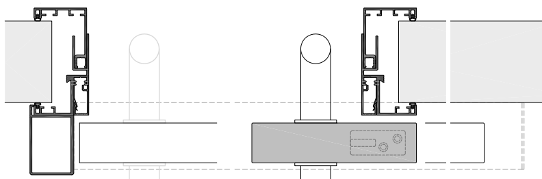
EUROKSV mit Auflaufprofil, Einzugsdämpfer optional
