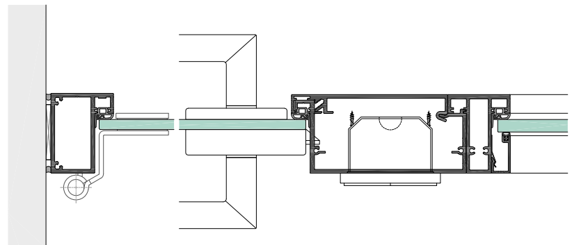
BS48-5-8G mit Ganzglastür und Glasseiteil, Pfosten KLS48-20 und integriertem Türterminal TTM
