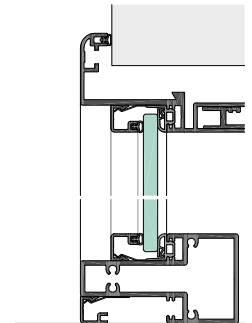
EURORSF48-5-8G Festverglasung, Kämpfer KST48
