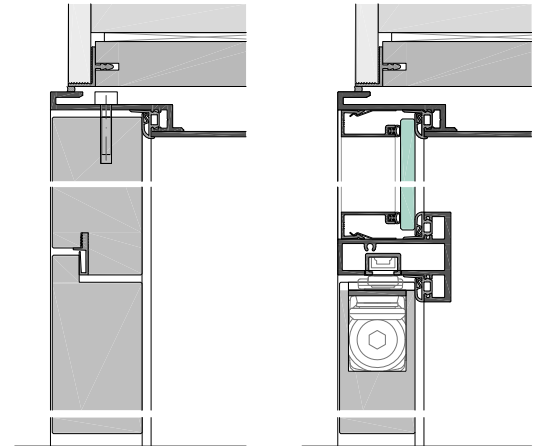
FZS56-V-5-50S mit Oberblende gegengefäلت
