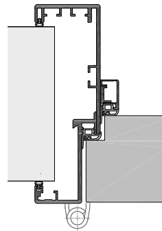
USTB48-5-70SL-ZAP als Doppelfalz zarge, Türblatt 70mm
