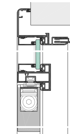
USTN48-5-42S mit Türblatt 42mm, Oberlicht, Kämpfer KLS48-20 sowie ITS
