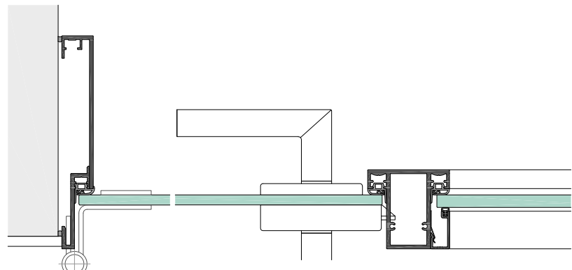
FZS48-V-5-8G mit Ganzglastür und Glasseiteil, Pfosten KLS48-35
