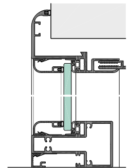
URS48-5-8G Festverglasung, Kämpfer KST48
