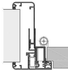
EURORF30-TH-50SL Turnhallenzarge mit Türblatt 50mm
