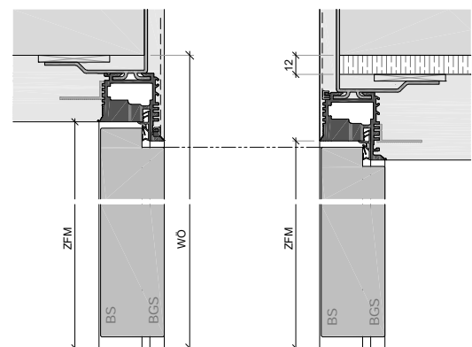
TZL / TZLI - abweichende Wandöffnung Nebeneinander angeordnete Elemente, mit unterschiedlichen Öffnungsrichtungen erfordern eine Differenz im Zargenfalzmaß von 12mm in der Höhe.
