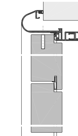
EUROFIS48-5-57SL mit Türblatt und Oberblende gegengefälzt
