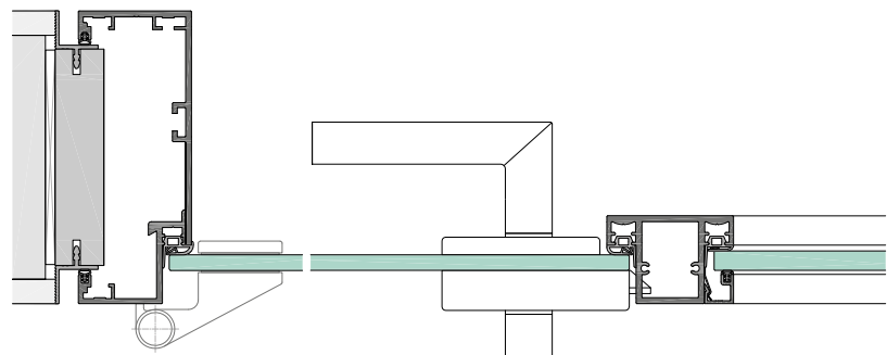
UFBV30-G-5-8G mit Ganzglastür 8mm, Pfosten KLF30-35 und Glasseite teil
