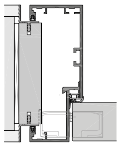
USBV48-G-5-42S mit verdecktem Bandsystem
