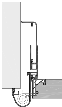
EUROFIS48-E-5-42S mit Fingerschutztürblatt 42mm
