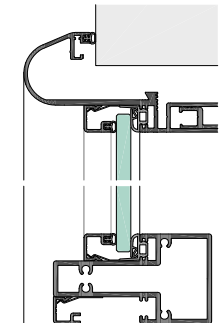
EUROFIS48-5-8G Festverglasung mit 8mm Glas, Kämpfer KST48
