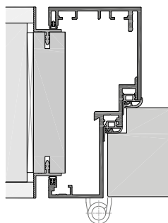
USDBV56-G-5-70SL Doppelfalz zarge mit 70mm Türblatt
