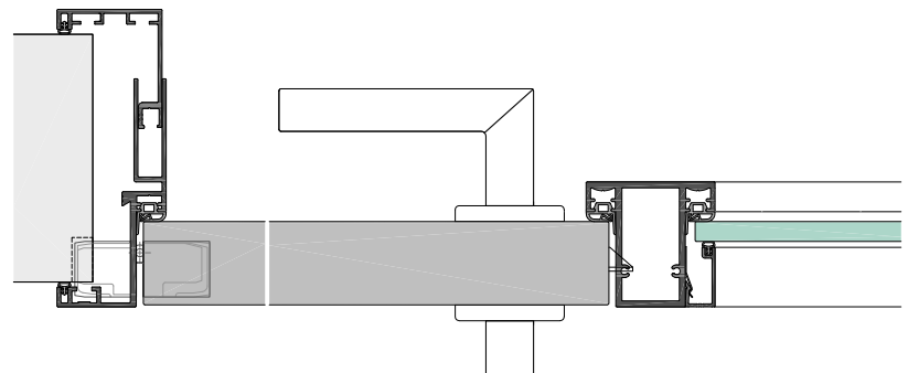
EUROKS48-5-42S Umfassungszarge mit Türblatt 42mm, sowie Glaseitenteil mit Pfosten KLS48-35
