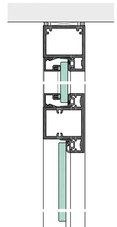
BF30-5-8G mit Ganzglastür, KLF30-35 und Oberlicht
