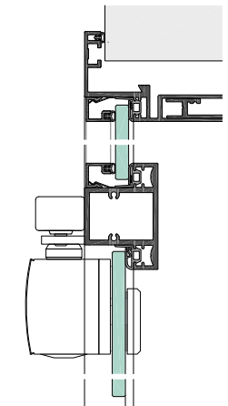
EUROKF30-5-8G mit Ganzglastür und Oberlicht, Kämpfer KLF30-35 sowie OTS
