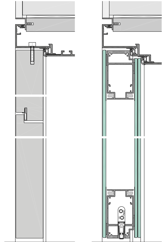
USBV56-G-5-50S Schattennutzarge mit 50mm Türblatt, Oberblende gegengefälzt
