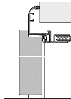
URF30-5-42F mit gefälztem Türblatt 42mm
