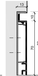
XN - Sockel zweiteilig bestehend aus Grund- und Deckprofil, mit Schattennut
