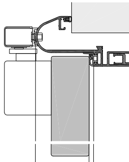
EUROFIS48-5-42S Türblatt 42mm, mit aufgesetztem Türschließer
