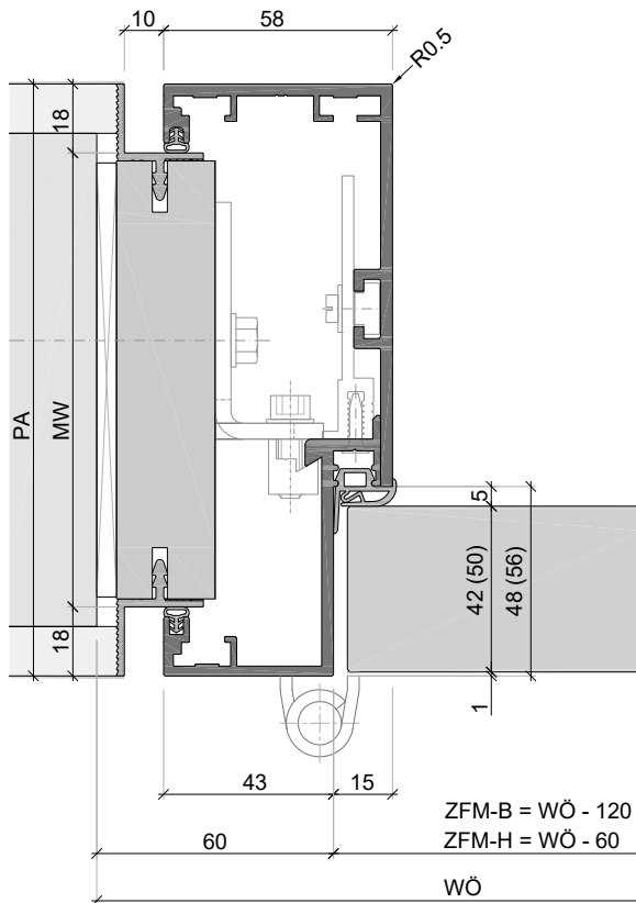
USBV48-G-5-42S (USBV56-G-5-50S) Umfassungszarge mit Grundzarge, Schattennut von 10mm, bündige Laibung, mit stumpf einschlagendem Türblatt
