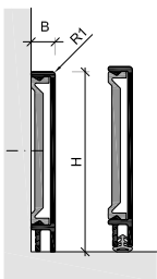
G - Sockel kantig, Montage mit Kunststoffclips
