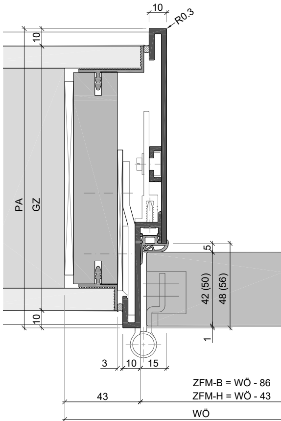
FZS48-V-5-42S (FZS56-V-5-50S) Laibungszarge mit 10mm Überstand, Türblatt stumpf einschlagend
