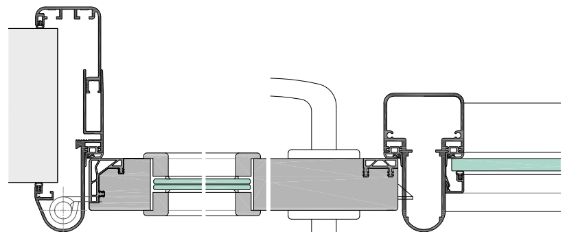
EUROFIS48-5-42S mit KFI mit Fingerschutztürblatt FST inkl. Lichtausschnitt, Pfosten KFI und Glasseiteeil
