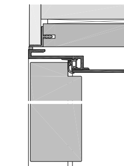
FZS48-5-60SL mit Türblatt 60mm stumpf mit Laibungsfalz
