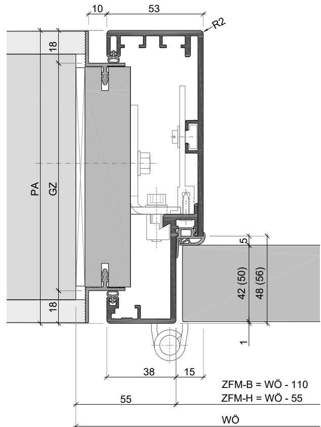
USTB48-G-5-42S mit Grundzarge und 10 mm Schattennut und stumpf einschlagendem Türblatt 42mm
