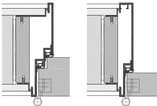
FZDS56-V-5-70SL Doppelfalz zarge mit Türblatt 70mm
