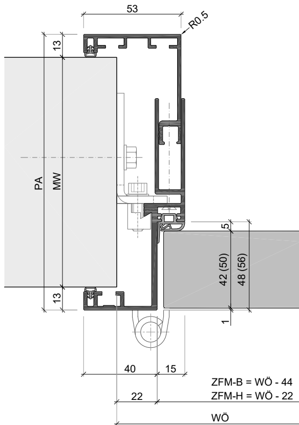
EUROKS48-5-42S (EUROKS56-5-50S) Umfassungszarge mit stumpf einschlagendem Türblatt
