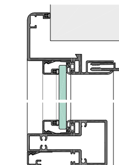
USTN48-5-8G Festverglasung, Kämpfer KST48
