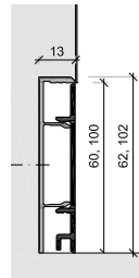
X - Sockel zweiteilig bestehend aus Grund- und Deckprofil
