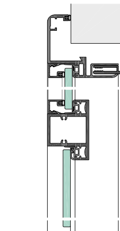
UNFN30-5-8G mit Ganzglastür 8mm, Oberlicht und Kämpfer KLF30-35
