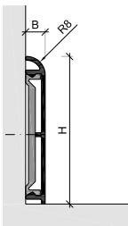
GR - Sockel gerundet, Radius 8mm, Montage mit Kunststoffclips
