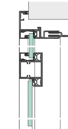
UNF30-5-8G mit Ganzglastür 8mm, Oberlicht und Kämpfer KLF30-35
