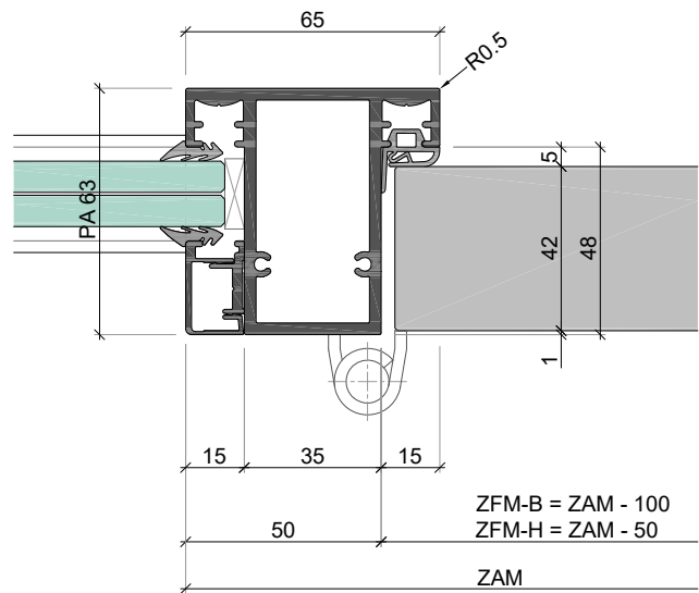
KLS48-35-5-42S Türblatt 42mm, in Glaswand integrierte Zarge mit Glasaufnahmeprofil GAP60
