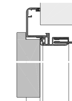
UNFN30-5-42F mit gefälztem Türblatt 42mm
