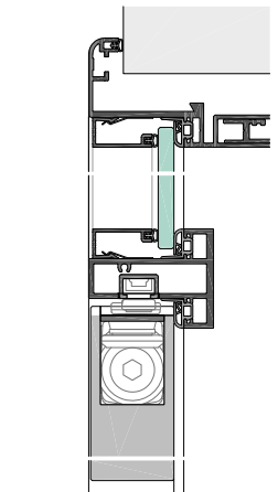
EURORS48-5-42s mit Türblatt 42mm und Oberlicht, Kämpfer KLS48-20 sowie ITS
