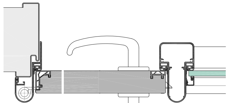
EFI48-5-42S mit KFI48
