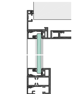
EUROKFF30-5-8G Festverglasung, Kämpfer KLF30-20
