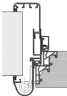
EUROFIS48-5-70SL-ZAP mit Fingerschutztürblatt FST 70mm
