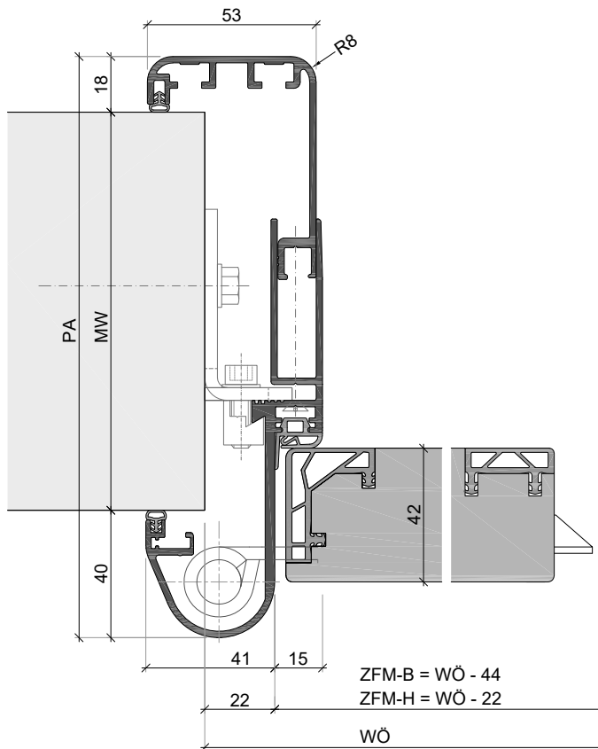
EUROFIS48-5-42S Umfassungszarge mit Fingerschutztürblatt FST
