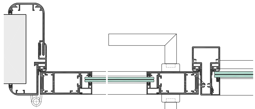
URS48-5-42S Element mit Aluminium-Rahmentür ART42, Pfosten KST48 und Glasseiteil
