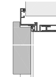
EUROKF30-5-42F mit gefälztem Türblatt 42mm
