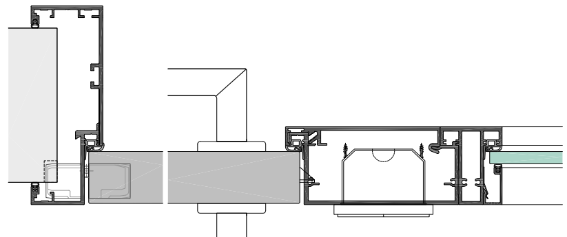
USBV48-5-42S mit verdecktem Bandsystem, Türterminal TTM, Pfosten KLS48-20 und Glasseitenteil
