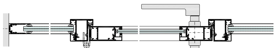
Glasaufnahmeprofil GAP60 mit Türzarge KLS48-35 und Rahmentür ART42
