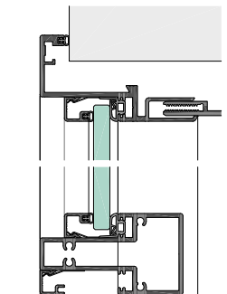
USTF48-5-8G Festverglasung mit Kämpfer KST48
