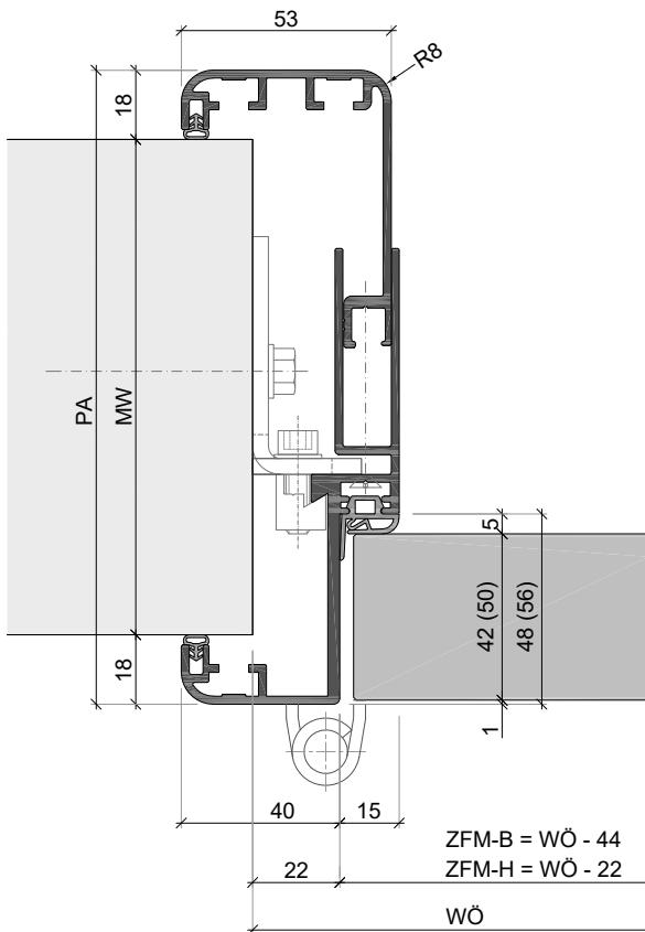
EURORS48-5-42S (EURORS56-5-50S) Umfassungszarge mit stumpf einschlagendem Türblatt
