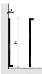
B - Winkelprofil mit Schenkel, Klebmontage
