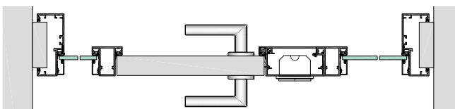
Umfassungszarge USBV48-G mit Grundzarge, Pfosten KLS48 und Türterminal TTM
