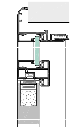
URS48-5-42S mit Türblatt 42mm und Oberlicht, Kämpfer KLS48-20 sowie ITS
