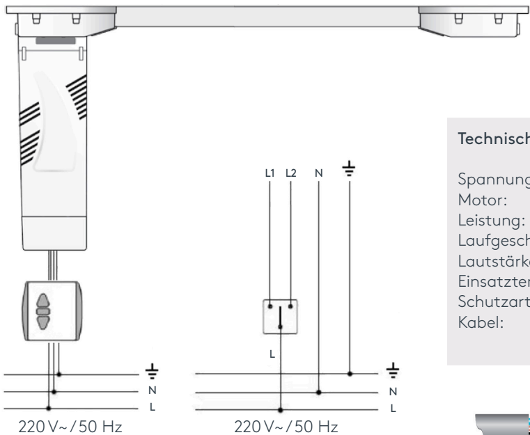
Farben Motorkabel
