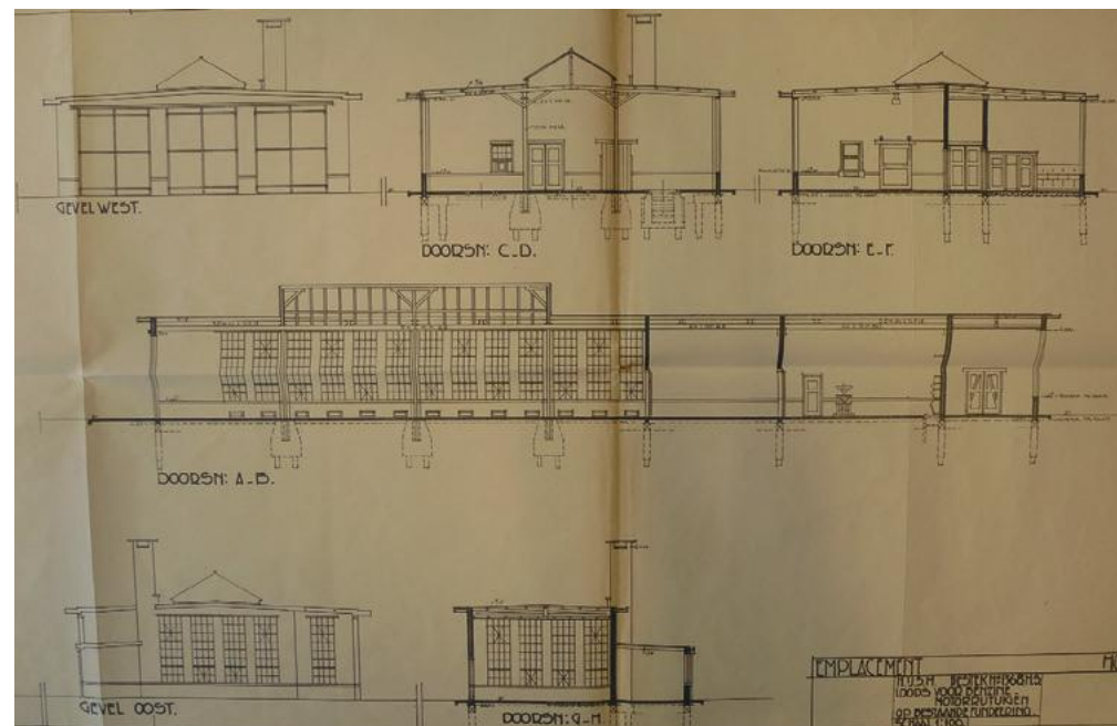
Voor- en achtergevel en doorsneden diesellocomotievenloods, 1929.
