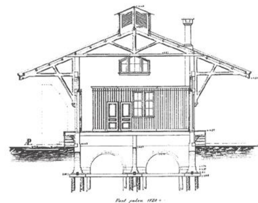
DOORSNEDE C. D.
