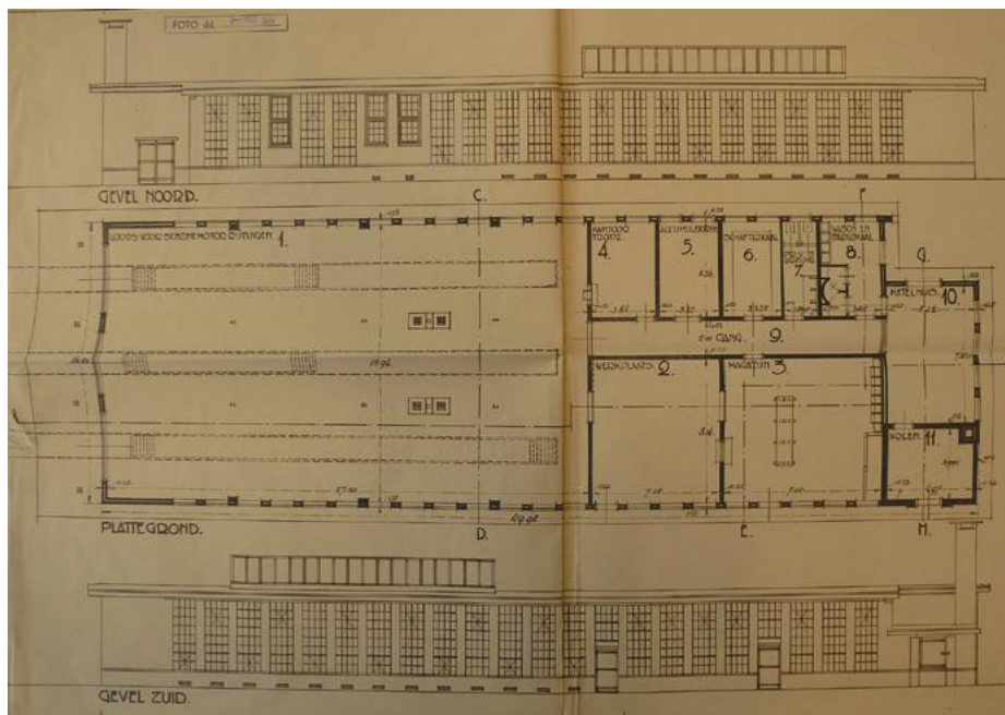
Plattegrond en zijgevels diesellocomotievenloods, 1929. [HUA]
