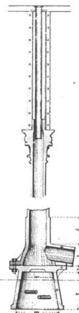
DOORSNEDE KOLOM.
