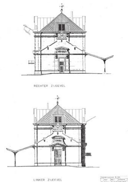
Zijgevels, nieuwe toestand, 1990 [HUA]
