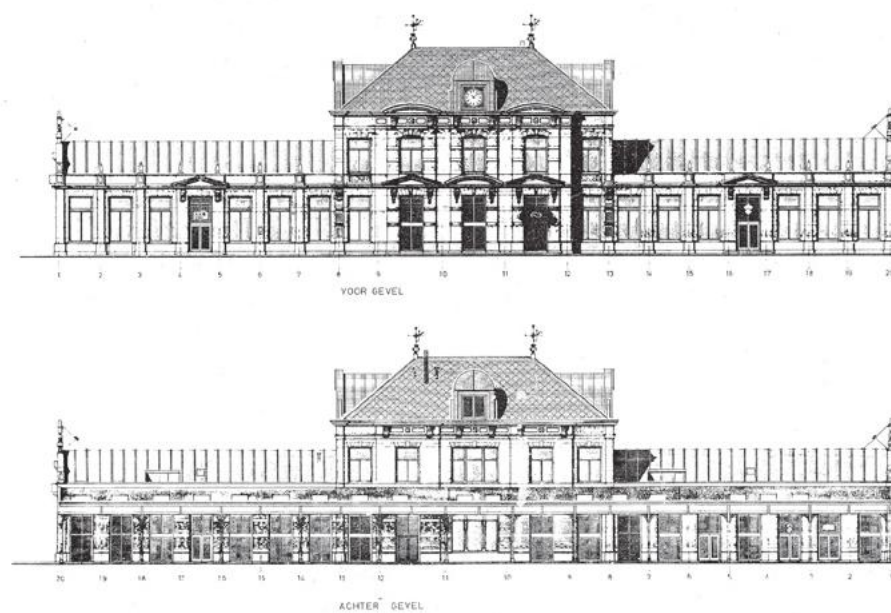
Voor- en achtergevel, nieuwe toestand, 1990 [HUA]
