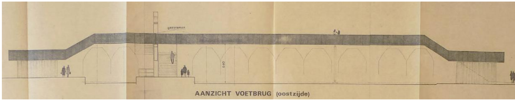
Aanzicht voetgangersbrug oostzijde en opgang zuidzijde, 1982. Architect K. van der Gaast [HUA]
