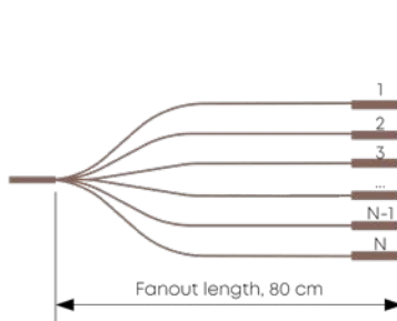
Fanout type 5
