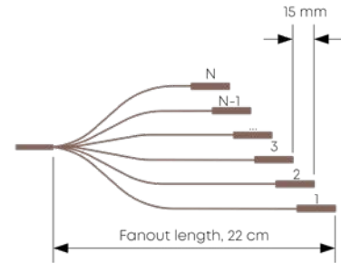
Fanout type 3
