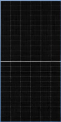
JAM72D40 LB 615W 2333 x 1134 x 30 32.5kg 144(6x24) 720 pcs
