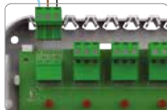
ДВУХПОЗИЦИОННЫЙ РЕГУЛЯТОР ДКЛЮЧЕНИЕ КОНТАКТА NO-COM
