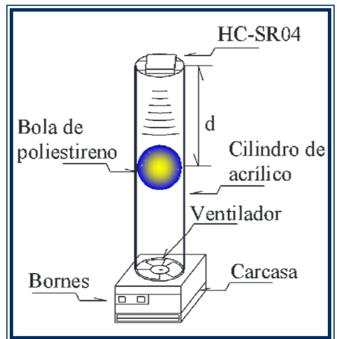
Fig. 1. Imagen del levitador neumático
