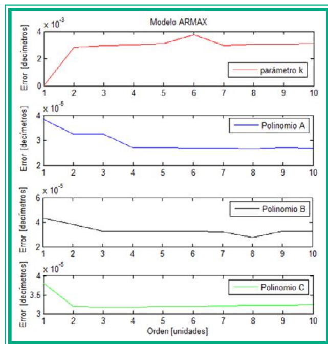
Fig. 6. Gráficas para la estructura del modelo ARMAX.
