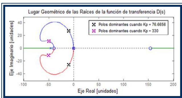
Fig. 11. Comparativo del LGR cuando K_p=76.6656 vs K_p=330
