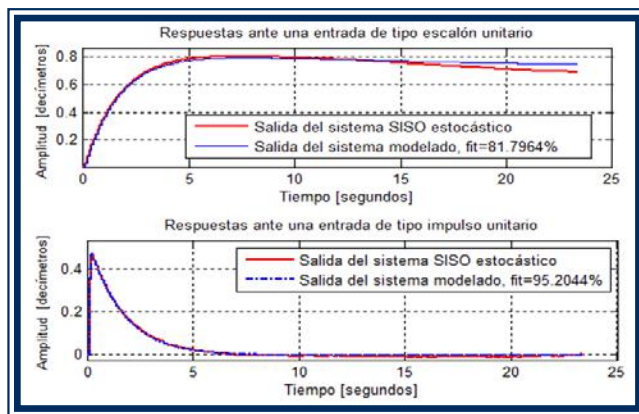
Fig. 13. Respuestas del sistema ante una entrada tipo escalón e impulso unitario.
