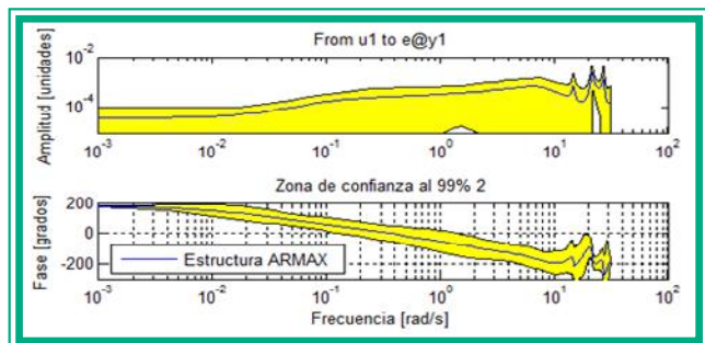
Fig. 16. Respuesta en frecuencia de la estimación realizada con el Modelo ARMAX.
