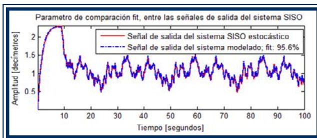
Fig. 17. Parámetro de comparación fit entre señales.
