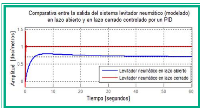
Fig. 10. Comparativa de la salida del sistema levitador neumático (modelado) en lazo abierto vs lazo cerrado controlado por un PID.
