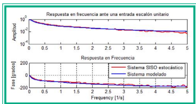
Fig. 14. Respuesta en frecuencia del sistema ante una entrada escalón: amplitud y fase.
