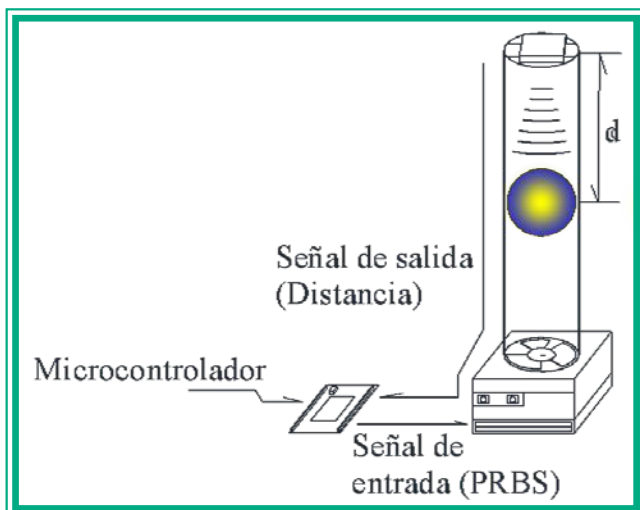
Fig. 2. Imagen del levitador neumático.
