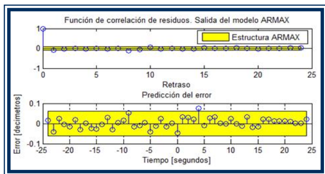
Fig. 15. Función de correlación de residuos usando el modelo ARMAX.
