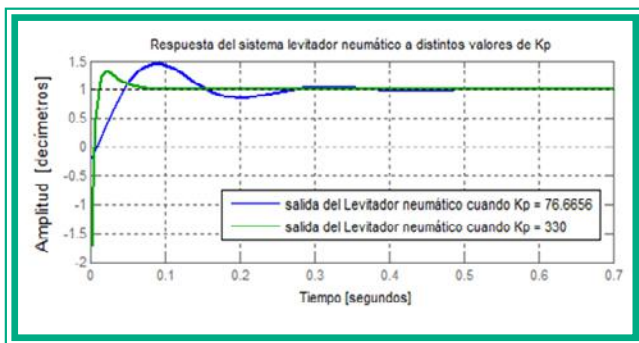
Fig. 12. Comparativa de la salida del sistema levitador neumático (modelado) a distintos valores de K_p .
