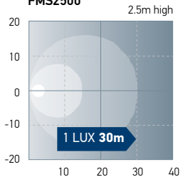
FMS2500
