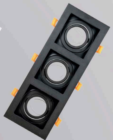
EM7003N. 3xGU10, 100x270mm. Metal. Orientable. Negro.
