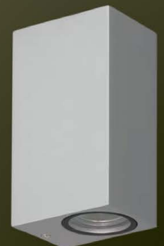
K1301G. Aluminio. 2×GU10. 16×7×7,5cm. Gris. IP54.
