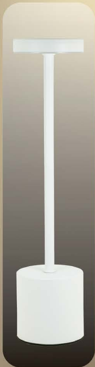
TL9001-BLANCO. LED 3W. Dimenzable. USB-C. 3000/4000/6500K Variables. Ø8x34cm. Blanco.
