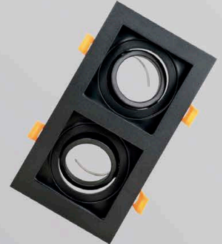
EM7002N. 2xGU10, 100x185mm. Metal. Orientable. Negro.
