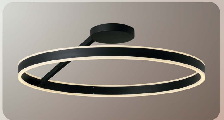
L7477N. LED 77W 3000/4000/6000K Variables. Ø50×16,5cm. Negro.
