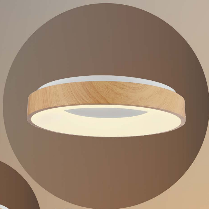
L4436. LED 36W. 3000/4000/6500K Variables. Ø50×9cm. Símil Madera.
