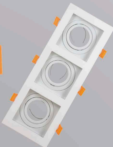
EM7003B. 3xGU10, 100x270mm. Metal. Orientable. Blanco.
