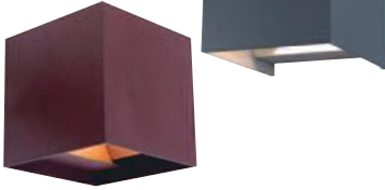
APLIQUE EXTERIOR OPEN LED COB 2X5W 700 LM 4000K IP54 1015019 BLANCO 1015020 ANTRACITA 1015020 ÓXIDO 24'95
