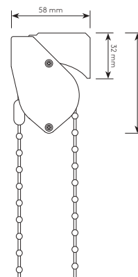
Querschnitt ISI-PIN mit Universalträger 45 mm
