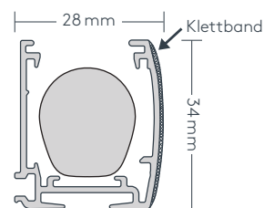
Querschnitt PowerView
