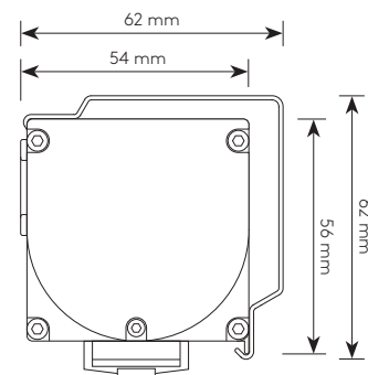
Querschnitt X-LARGE Elektro
