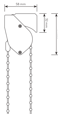
Querschnitt ISI-CLICK mit Universalträger 45 mm
