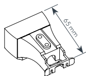
Wandträger 65 mm (ohne Aufzählung) Art. Nr. 9430-12
