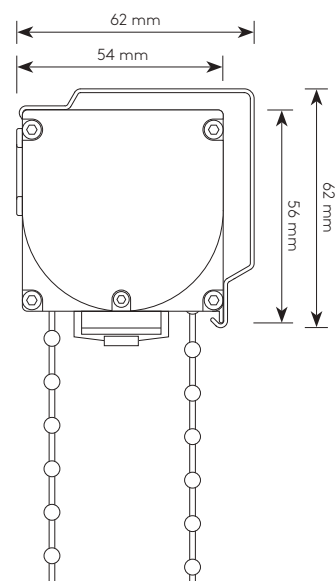
Querschnitt X-LARGE
