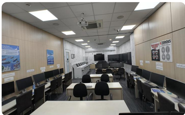
Kongsberg Full Mission LNG Simulator
