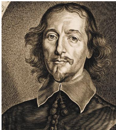
Das Vakuum Der Experimentalphysiker und Bürgermeister Otto von Guericke entdeckte die gewaltige Kraft des atmosphärischen Luftdrucks, nebenbei erfand er die Luftpumpe.
