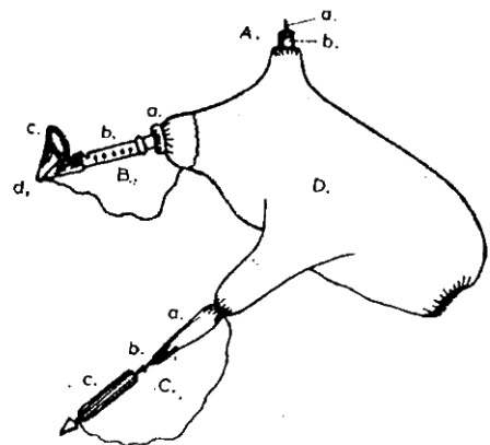
Cimpoiul și părțile sale: A. suflaciu , alcătuit din a) cartuș de alamă, b) inel de lemn ferecat cu alamă; B. carabă , alcătuită din a) bucea, b) carabă, c) lulea, d) răsunătoare; C. bizozi , alcătuit din a) soc, b) mijlocariu, c) bizozi; D. burduf .
