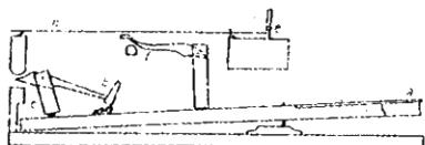
Mecanismul pianului (fig. 1): a) clapă (tastă), b) ciocânel, c) sistem de pîrghii pentru acționarea ciocânelului, d) coardă, e) cui pentru fixarea și acordarea corzii, f) sistem de estompare a vibrațiilor corzii.
