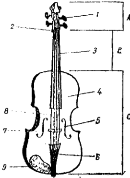
Violină (fig. 1). Părți componente: A. capul violinei; B. gîtul violinei; C. corpul violinei: 1. culele, 2. prăgușul, 3. limba, 4. cutia de rezonanță, 5. efurile, 6. cordarul, 7. călușul, 8. corzile, 9. bărbia.
