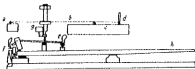
Mecanismul pianului (fig. 2): a) placă de rezonanță (pe care se fixează o extremitate a corzii), b) coardă, c) pragul cutelor, d) cui (folosit la acordaj), e) ciocânel, f) sistem de pîrghii care acționează ciocânelul, g) sistem mecanic de variație a intensității sunetului prin oprirea sau prelungirea vibrațiilor, h) clapă (tastă).
