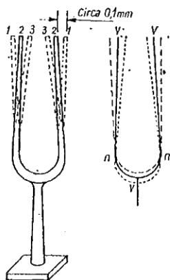
Vibrație. Parcurgând simultan drumurile 1-2-3-2-1, brațele diapazonului efectuează o vibrație completă. În n (nod) metalul nu vibrează, iar în v (ventru) amplitudinea de vibrație este maximă.
