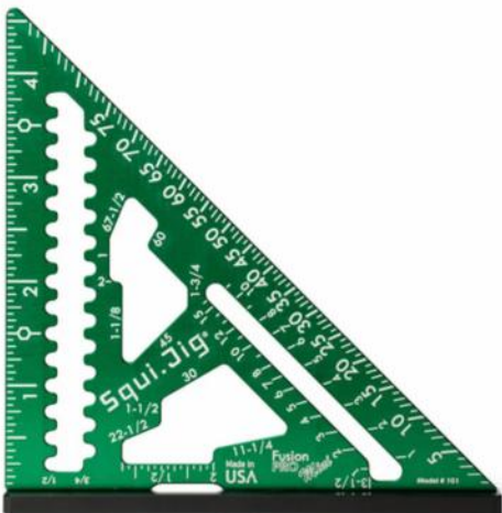
Fusion 4.5 inch Mini Pro Square - 3/16" Heel Colour: Green (FP45Green316)
