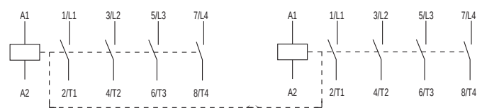
Ex9CDR... 4P 4NO
